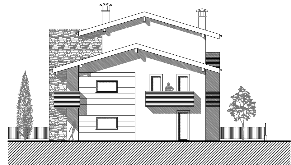
PROSPETTO NORD
